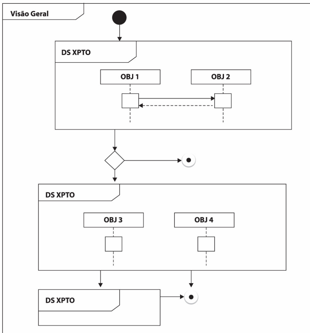
Figura 16.1 Diagrama de interação – Visão Geral.
